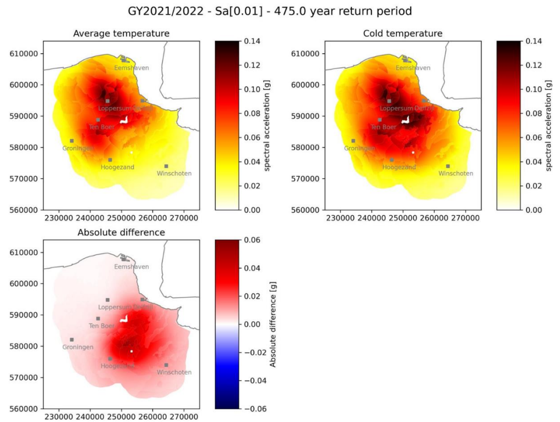
Figuur 4.4 Absolute verschil in jaarlijkse seismische dreiging bij een herhalingsjijd van 475 jaar tussen een koud en een gemiddeld temperatuurverloop voor gasjaar 2021/2022.
