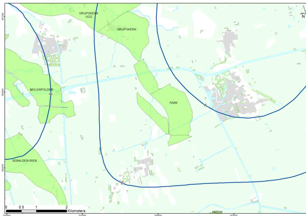
Figuur 7-6: Prognose voor 2050 van de totale bodemdaling door gaswinning voor het Faan voorkomen in combinatie met naburige voorkomens 22 jaar na beëindiging van de winning in Faan. De contourlijnen geven de voorspelde bodemdaling in cm aan.
