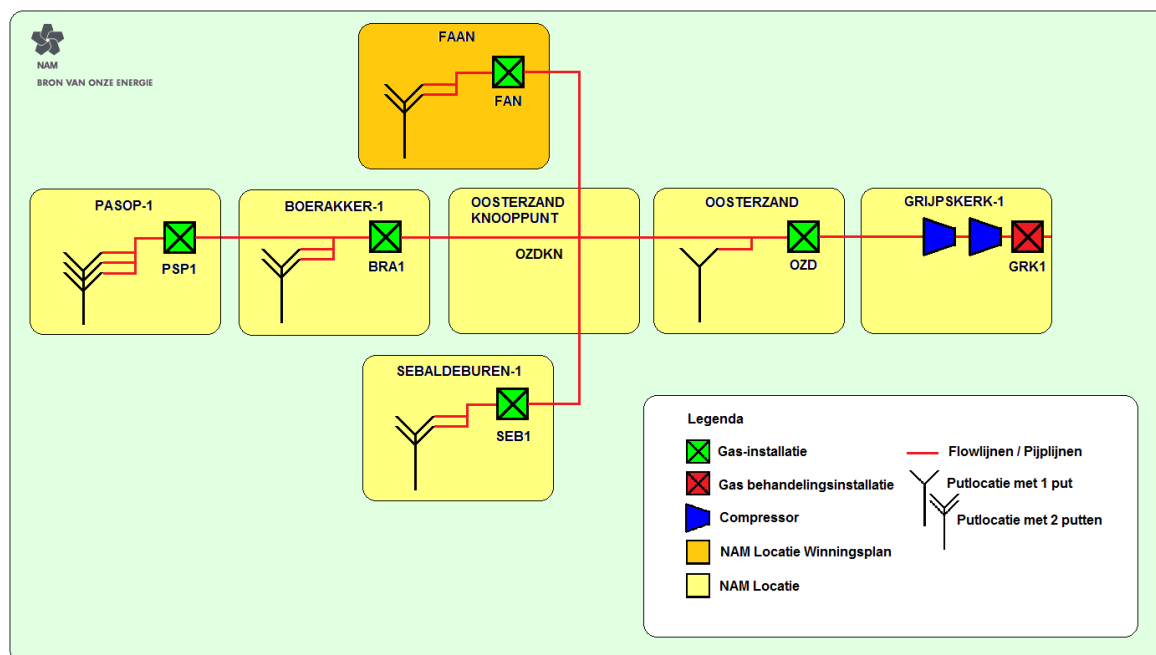
Figuur 3-3: Schematische weergave gasbehandeling en afvoer
