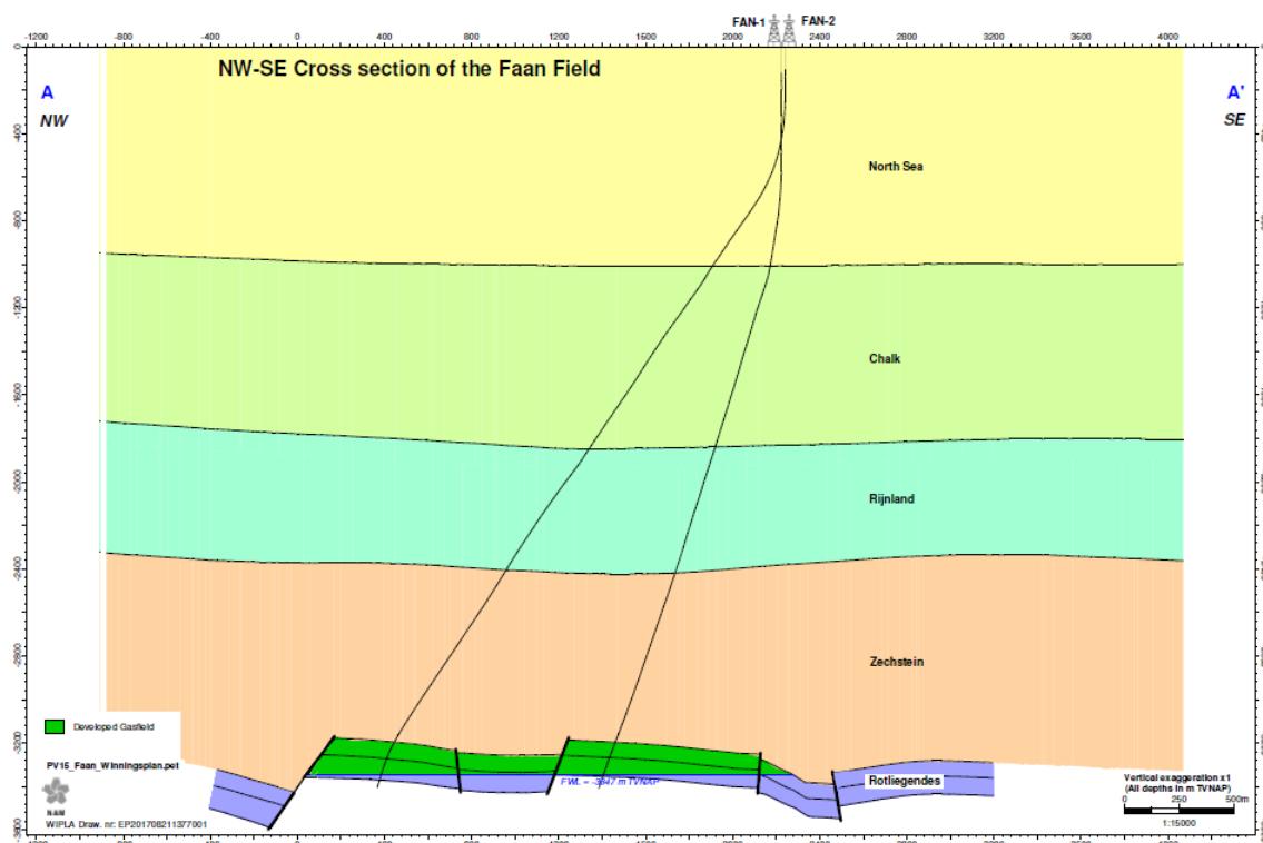
Figuur 5-1: Dwarsdoorsnede van maaiveld tot aan het reservoir over het Faan voorkomen.
