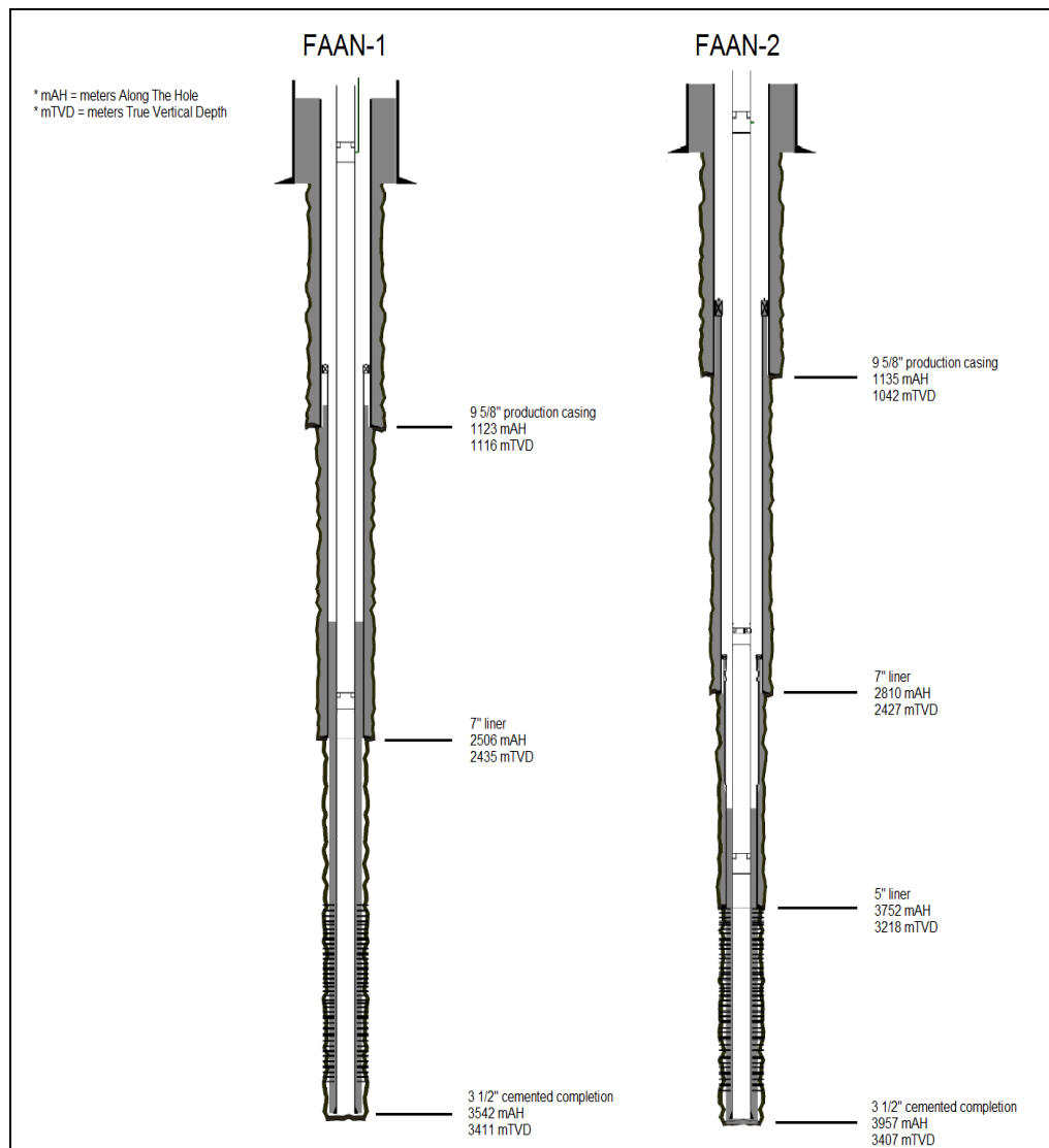
Figuur 4-3: Schematische voorstelling van de putverbuizingen in Faan. Dieptes zijn aangegeven langs de put (in meter "along hole", mAH en meter "True Vertical Depth", mTVD). Aangezien de put gedeveerd is geboord, is de verticale diepte t.o.v. NAP (mTVD) altijd minder dan de 'along hole' diepte (mAH)
