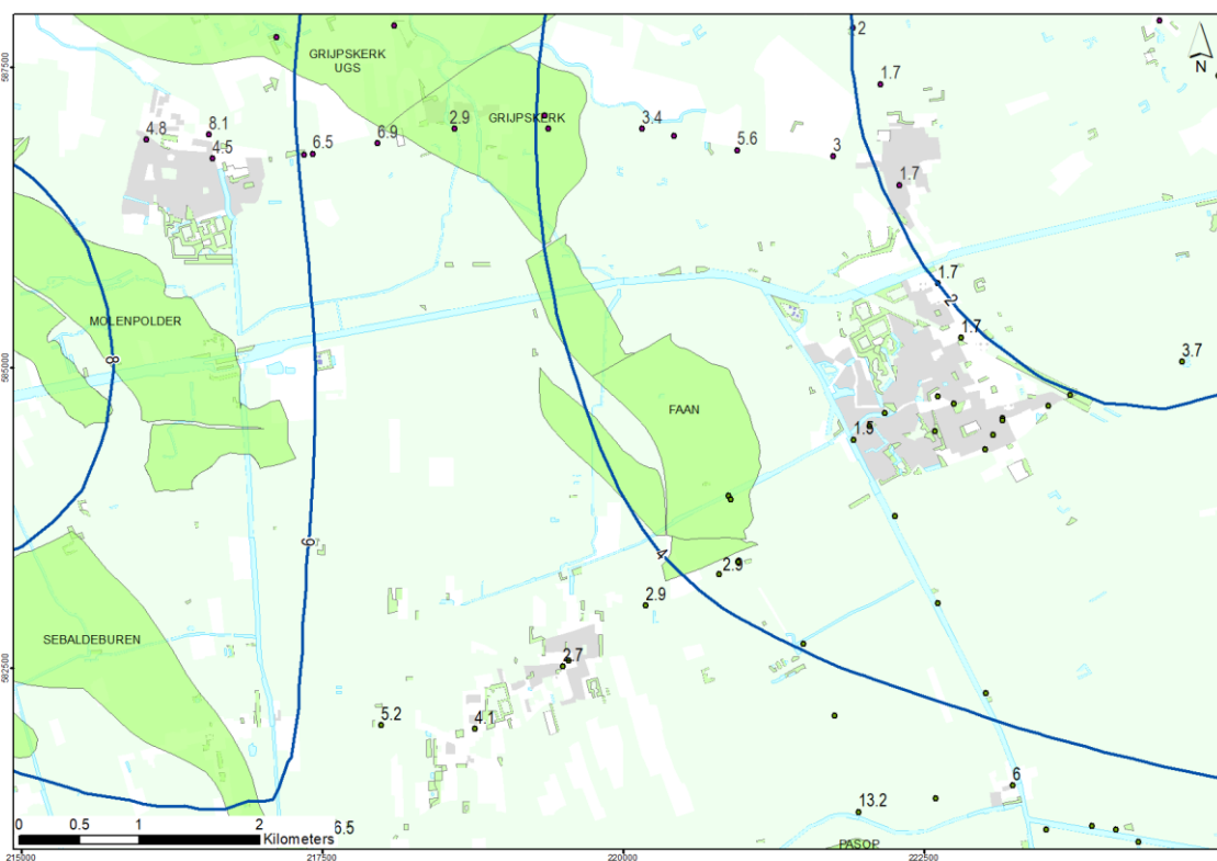
Figuur 7-3: In 2018 gemeten bodemdaling sinds de nulmeting in 1987 weergegeven op de peilmerken (punten). De contouren geven de gemodelleerde bodemdaling in cm.
