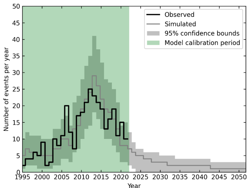
Figuur 7.1 Verwachte seismische activiteit en variatie per gasjaar volgens de aanbevelingen uit sectie 7.1. Zie Figuur 3.1 voor het onderschrift.
