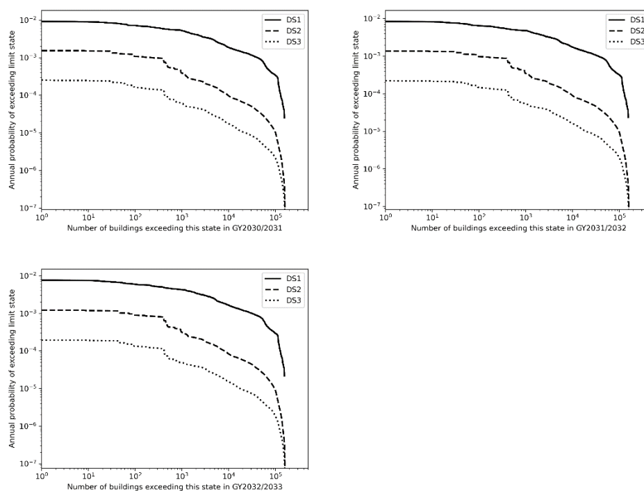
Figuur 6.1 Jaarlijkse overschrijdingskans voor schadetoestanden DS1 t/m DS3 voor gasjaar 2022/2023 tot en met gasjaar 2032/2033 voor alle gebouwen in de exposure database.
