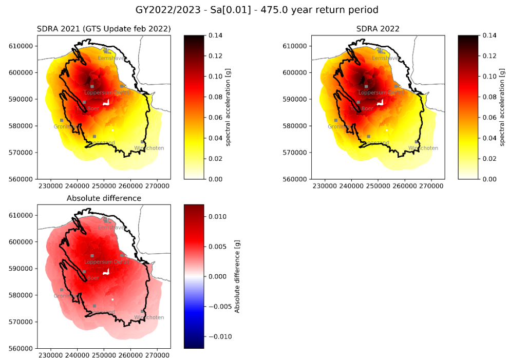
Figuur 7.2 Absolute verschil in jaarlijkse seismische dreiging bij een herhalingsjijd van 475 jaar tussen SDRA 2021 (GTS-update februari 2022; zie TNO (2022b)) en de SDRA 2022 voor gasjaar 2022/2023 volgens de aanbevelingen uit sectie 7.1. De hernieuwde kalibratie van het seismologisch bronmodel leidt tot een toename van de seismische dreiging (tot 0,01 g) over de gehele gemodelleerde invloedssfeer van het Groningenveld.
