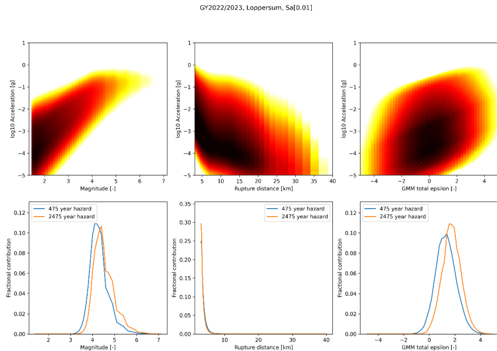
Figuur A.2 Disaggregatie van de seismische dreiging voor Loppersum. Zie Figuur A.1 voor het onderschrift.
