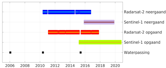
Figuur 1: Temporele bemonstering van satelliet opnames en tijdstippen van de waterpassingen.
