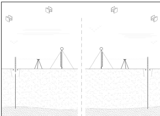
Figuur 1 Principeschets van de signaleringsmeting met als doel het meten van hoogteverschillen tussen de ondergrondse merken en de overige peilmerken op de 4 meetlocaties. De signaleringsmetingen bestaan uit GPS-metingen voor het bepalen van de hoogten (ETRS) van de ARP's van de meetpalen en uit waterpas-metingen om het hoogteverschil te bepalen tussen de peilmerken en de ARP's van de meetpalen.
