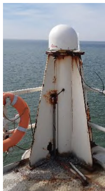
Figuur 5 Meetlocatie Zuidwal GPS-met een Leica AR25-choke ring antenne (meting mei 2022)
