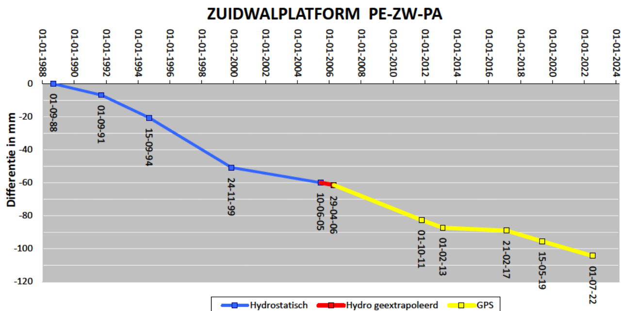
Grafiek 1 Gemiddelde differenties peilmerken 005C0022 en 005C0023
