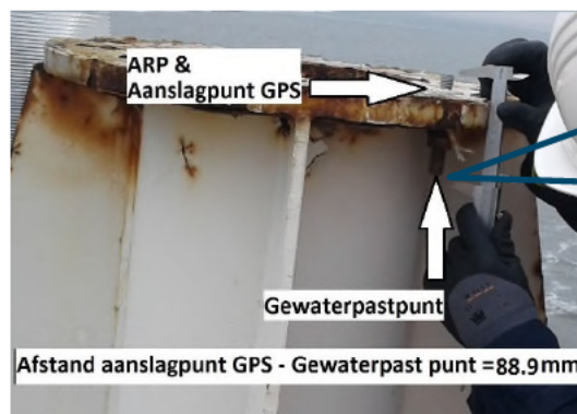
Figuur 12 Meetpunt voor de aansluitende waterpassing
