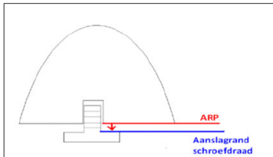
Figuur 10 Schets ARP/Aanslagrand
