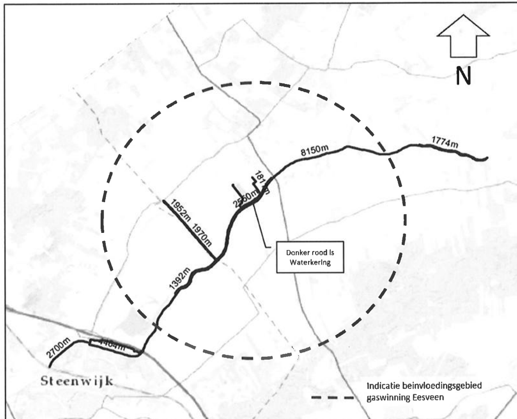
Figuur 1 : kaartbeeld waterkering op- en rond het voorkomen Eesveen
