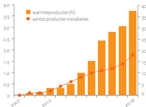
Totale aardwarmteproductie per jaar.
