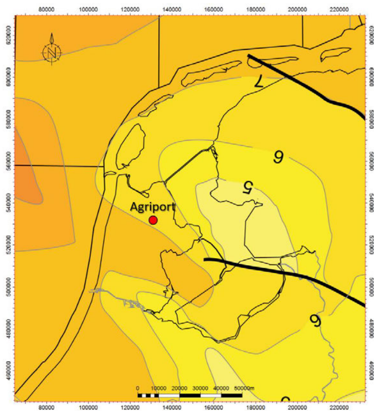
Figuur 27. Dieptecontouren voor Top Slochteren, met bijbehorend breukpatroon
