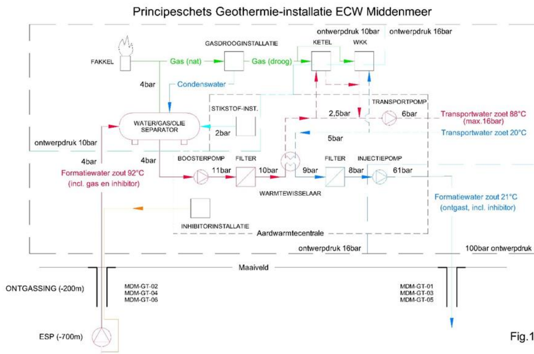
Figuur 7. Principe schets/ blokschema Geothermie-installatie ECW Middenmeer (is van toepassing op gehele installatie en 6 putten (winningsvergunning I en II).
