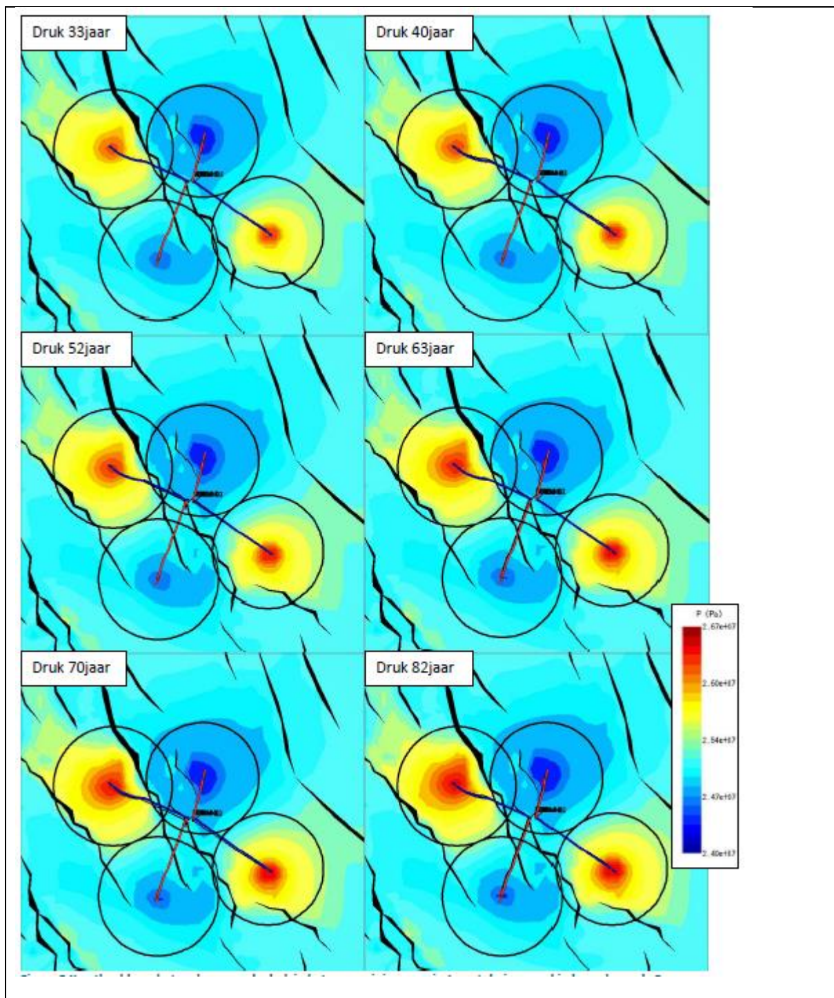
Figuur 23: Kaart met de drukverdeling in de aquifer bij winning. (de omhullende van de \pm 1 bar dP t.o.v. reservoir druk
