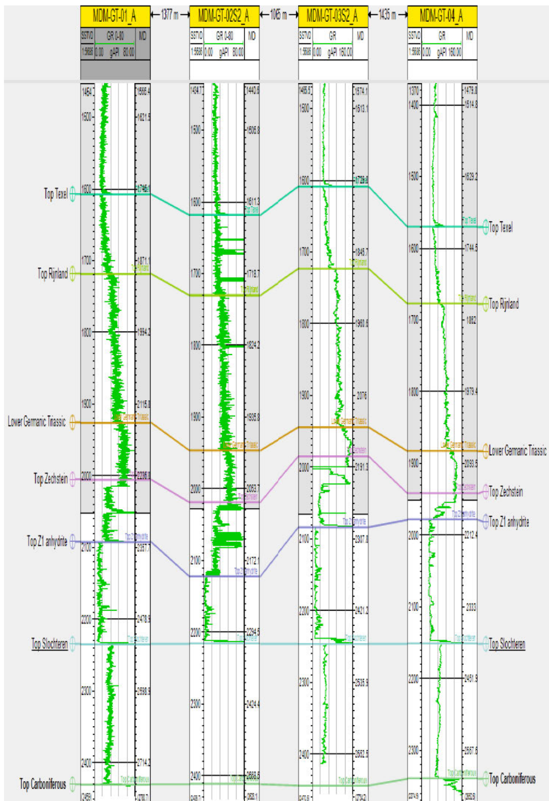
Figuur 20. Correlatiepaneel door putten MDM-GT-01 t/m MDM-GT-04.
