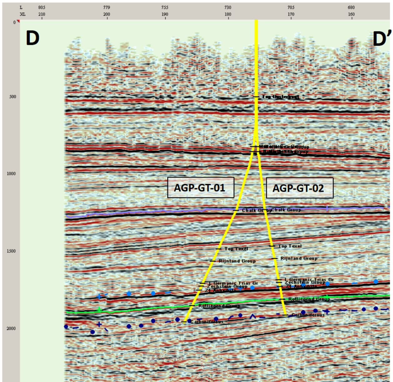
Figuur 16. Seismische sectie (sub-) parallel aan de dominante breuktrends.
