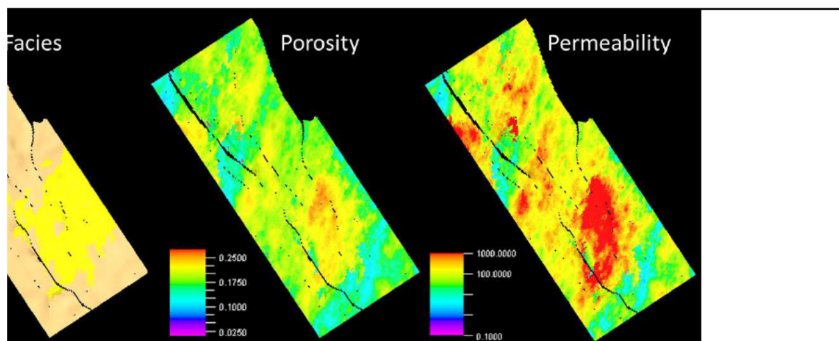
Figuur 21: Porositeit (links) en permeabiliteit (rechts) voor het Middenmeer gebied.
