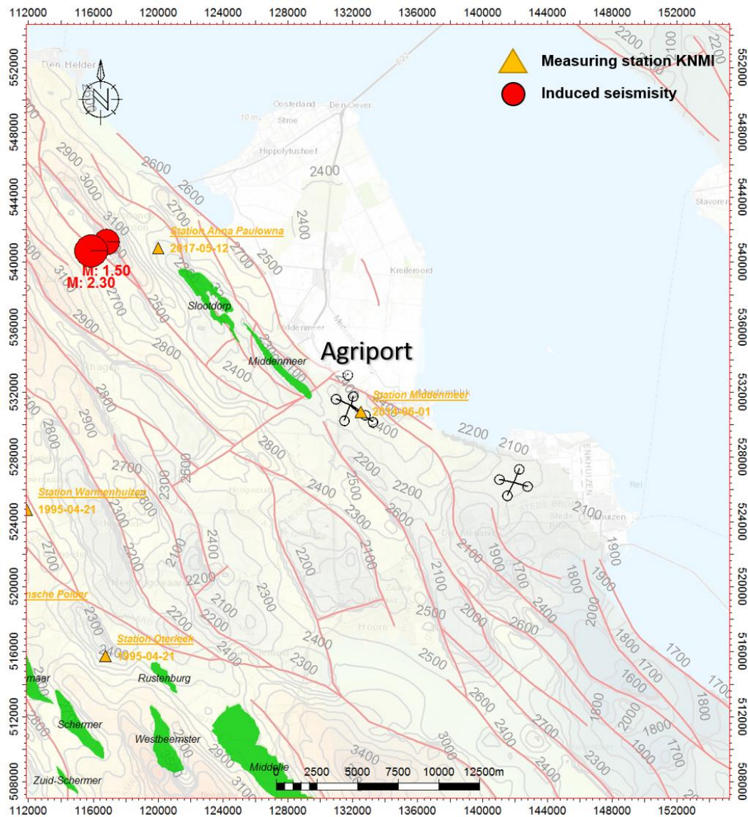
Figuur 31. Kaart met de seismische epicentra in het gebied. De rode cirkels geven geïnduceerde seismiteit aan. In het oranje de meetstations en ook zichtbaar top Slochteren met bijbehorende breuklijnen. Opgemerkt wordt dat er in het weergegeven gebied geen natuurlijke seismiteit is waargenomen.
