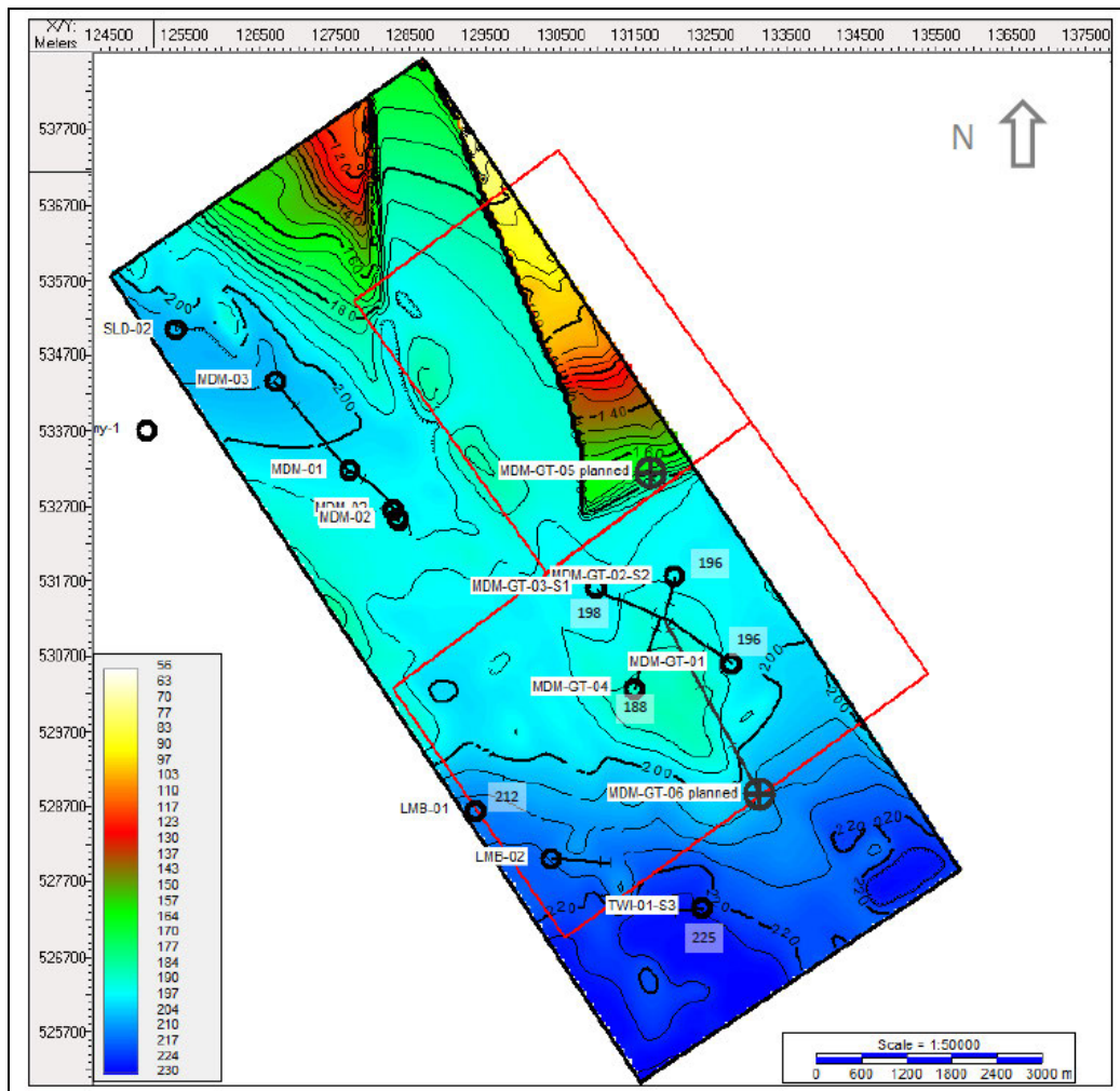
Figuur 18: Dikte voor Slochteren Zandsteen in het winningsgebied.
