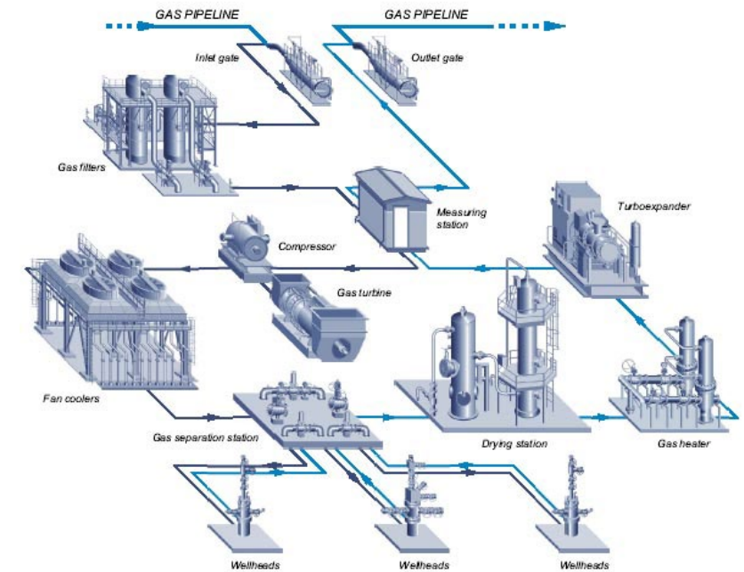
Voorbeeld van een gasbuffering keten. (bron: www.abb.com )
