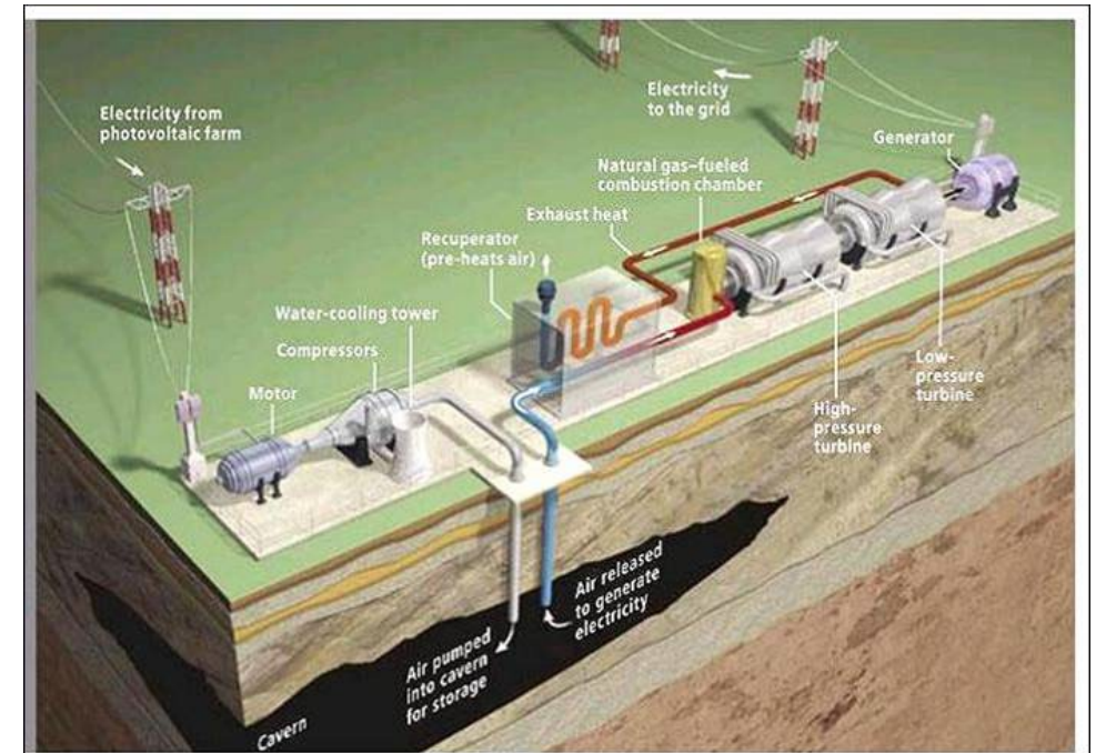
Schematisch overzicht van een perslucht opslaglocatie (bron: climatetechwiki.org)
