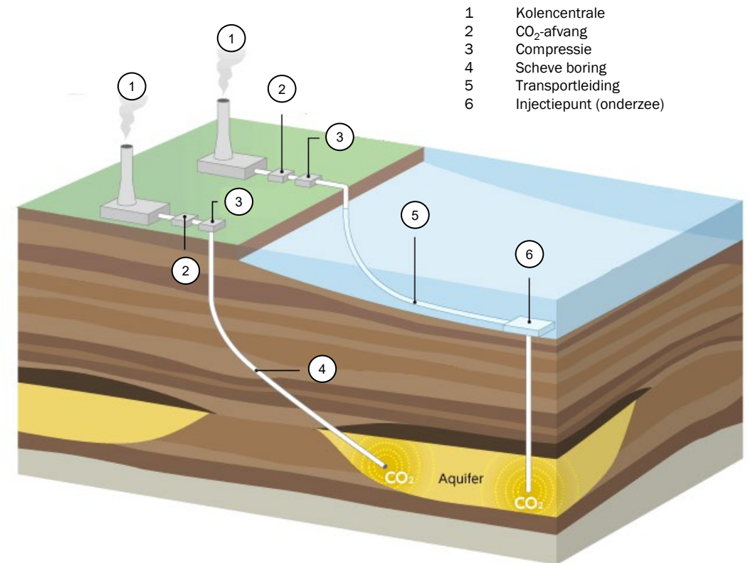
Voorbeeld van een CO 2 opslagketen. (bron: Japex)
