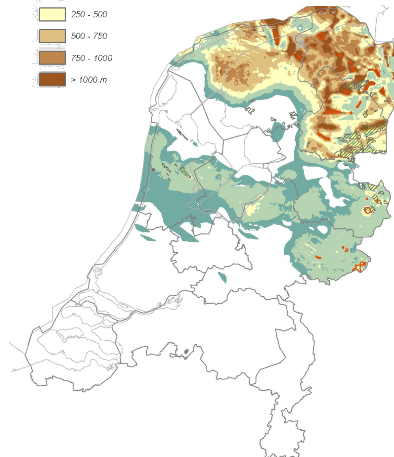
Verbreiding en dikte van steenzoutvoorkomens
