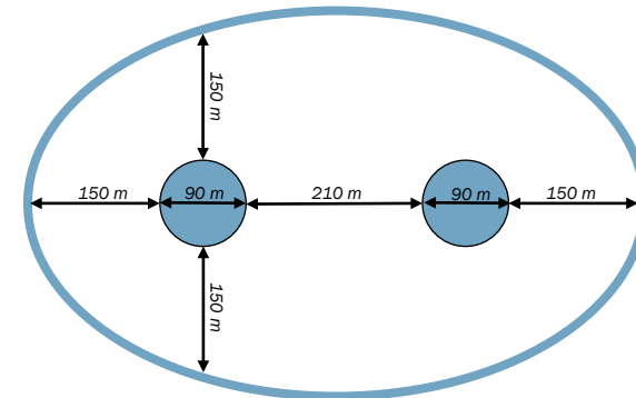
Dimensie en afstand tussen cavernes (bron: TNO, 2011)
