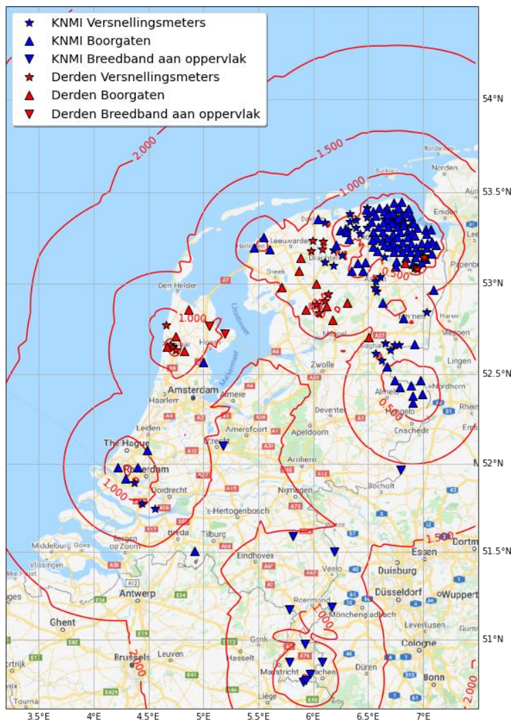
Figuur 1: Overzicht van de locatiedrempel in Nederland (status mei 2021) [1] . De driehoeken geven de locaties aan van de boorgatstations en de sterren van de versnellingsmeters. De De omgekeerde driehoeken tonen de breedbandstations.
