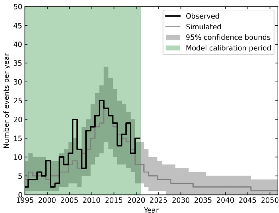
Figuur 3.1 Verwachte seismische activiteit en variatie per gasjaar voor het scenario GTS update februari 2022 . Op de horizontale as staat het kalenderjaar. Op de verticale as staat het aantal bevingen met een magnitude gelijk aan of hoger dan 1,5 opgeteld per gasjaar. De zwarte lijn geeft het aantal observaties in het verleden weer. De donkergrijze lijn geeft het verwachte aantal bevingen weer. De lichtgrijze band om de grijze lijn is de onzekerheidsband. Het groene vlak geeft aan dat het model gekalibreerd is op de periode tot 1 januari 2021.
