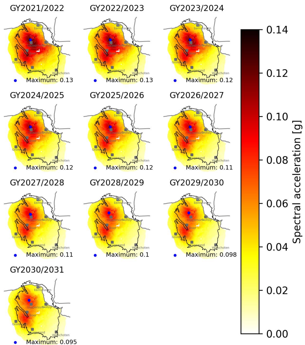
Figuur 4.1 Overzicht van de jaarlijkse seismische dreigingskaarten voor gasjaar 2021/2022 tot en met gasjaar 2030/2031 voor het scenario GTS update februari 2022 .
