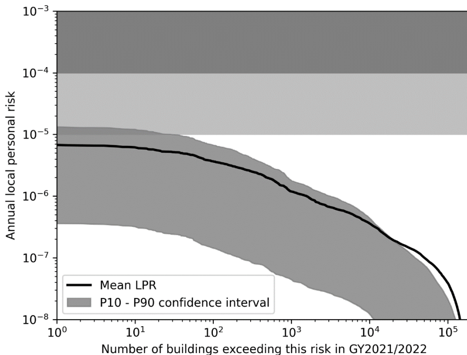
Figuur 5.1 LPR grafiek voor gasjaar 2021/2022 voor scenario GTS update februari 2022 . Op de horizontale as staat het aantal als onveilig te beschouwen gebouwen; op de verticale as het LPR. De grafieken geven voor elk aantal op de horizontale as de LPR waarde die door deze groep overschreden wordt. De dikke zwarte lijn geeft de verwachtingswaarde (mean) van het LPR aan. De donkergrijze band geeft de spreiding in uitkomsten van de beslisboom voor modelonzekerheden weer voor een betrouwbaarheidsinterval van tussen percentielen P10 en P90. De twee horizontale vlakken in lichtgrijs geven het tijdelijke ( 10^{-4} ) en permanente ( 10^{-5} ) LPR-niveau van de Meijdamnorm aan.
