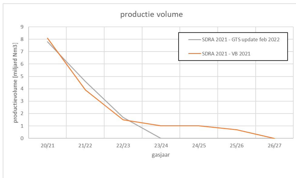
Figuur 2.1 Productievolumes cf. de initiële operationele strategie voor gasjaar 2021/2022 en verder (Vaststellingsbesluit 2021) weergegeven met de oranje lijn. De grijze lijn betreft de geactualiseerde GTS prognose (feb 2022) voor gasjaar 2021/2022 en verder.
