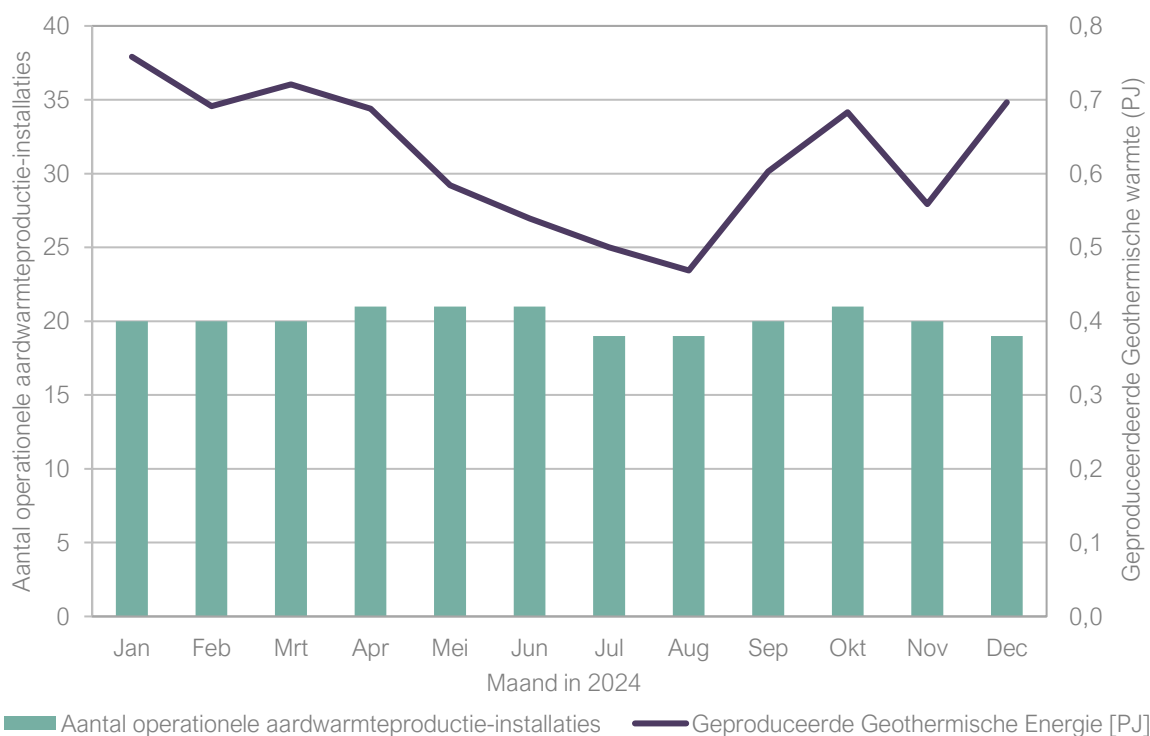
Figuur 5.2 Maandelijkse aardwarmteproductie in petajoules (PJ) in 2024 en het aantal aardwarmteproductiesystemen dat per maand heeft bijgedragen aan de gerapporteerde productie. NB: niet alle installaties zijn het volledige jaar operationeel.
