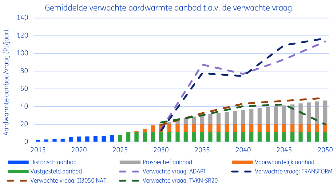
Figuur 6.1. Het historische en geprognosticeerde aardwarmte aanbod uitgezet tegen de verwachte vraag voor de periode 2015 – 2050. De historische productie is afkomstig uit het Jaarverslag Delfstoffen en Aardwarmte 2023 (Ministerie van Klimaat en Groene Groei, 2024). Het verwachte aanbod, onderverdeeld in 3 groepen, zijn stochastisch bepaald en in deze grafiek is alleen de P50 waarde weergegeven. Voor de verwachte vraag naar aardwarmte is gebruik gemaakt van de verschillende energiescenario's die geselecteerd zijn voor deze studie. Hierbij is gebruik gemaakt van een interpolatie tussen de verschillende datapunten.
