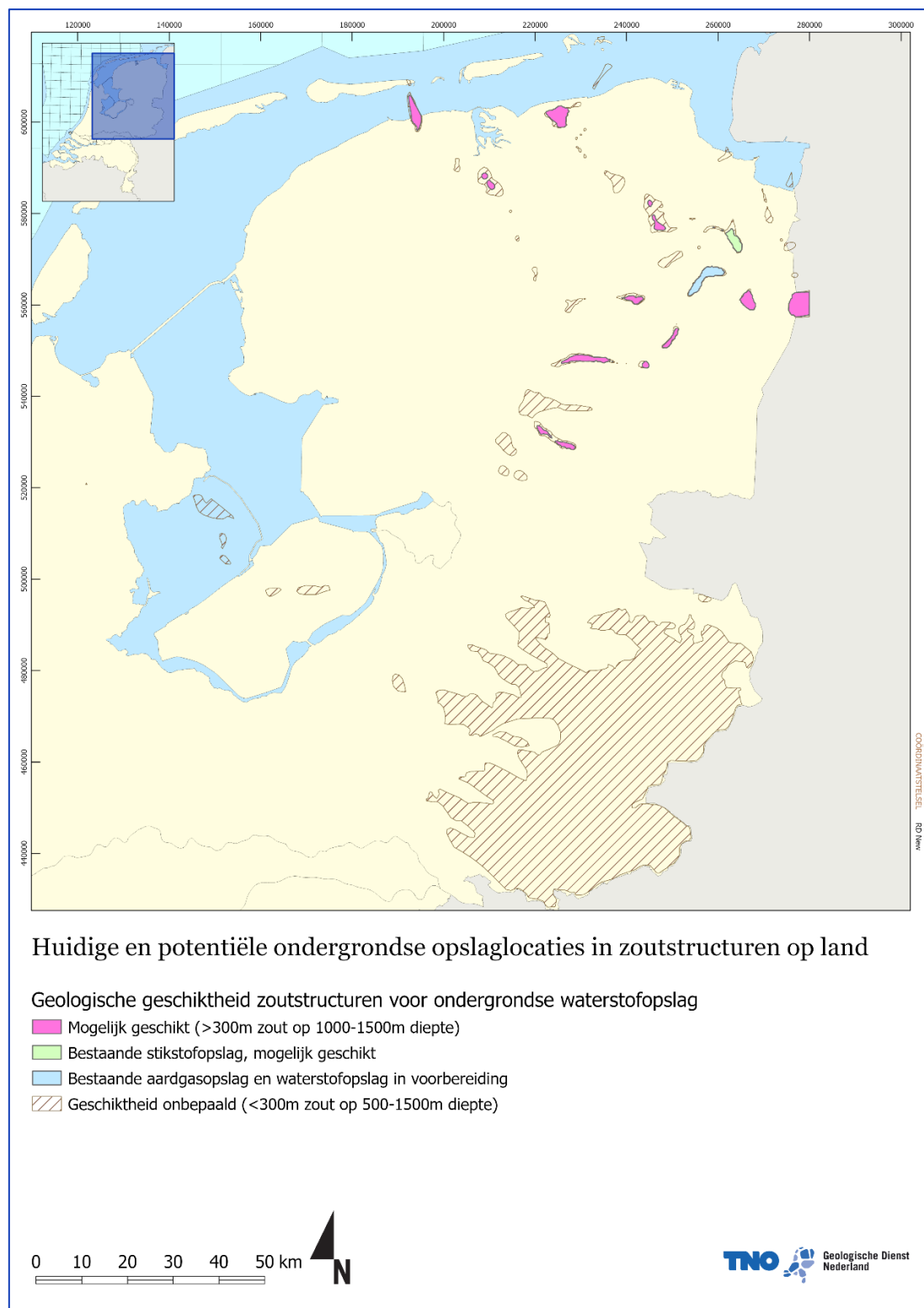
Figuur 8.4. Overzicht van mogelijk geschikte zoutvoorkomens en structuren voor aanleg van opslagcavernes.
