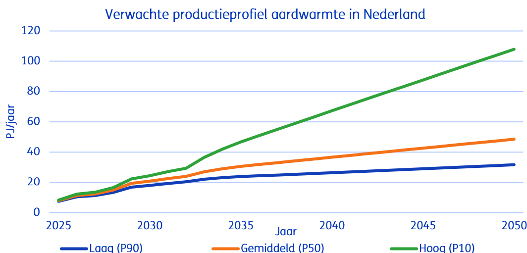
Figuur 6.5. Resultaat van de productievoorspelling voor aardwarmte in Nederland. Deze grafiek toont de gesommeerde productieprognoses uit de vastgestelde, voorwaardelijke en prospectieve aardwarmte voorraden. Gepresenteerd in P90, P50 en P10 uitkomsten.
