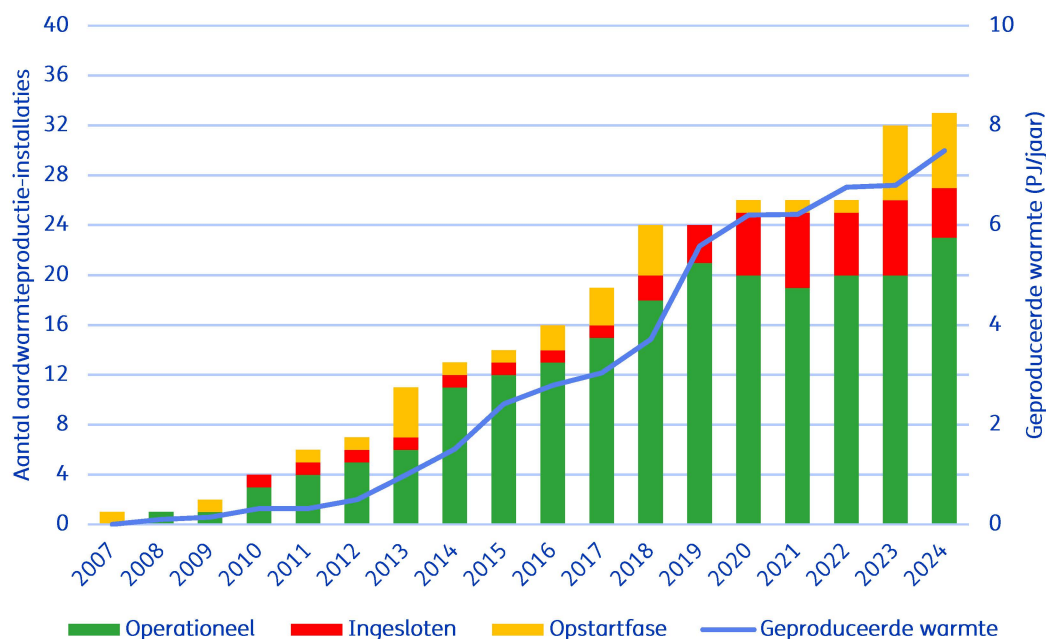
Figuur 6.3. Aantal aardwarmteproductie-installaties, onderverdeeld naar status operationeel, ingesloten en opstartfase, uitgezet tegen de jaarproductie aan aardwarmte (PJ/jaar). Tot en met 2013 is de jaarproductie afkomstig uit: Hernieuwbare energie in Nederland 2013 (CBS, 2014). Vanaf 2014 wordt de warmteproductie gerapporteerd in het Jaarverslag Delfstoffen en Aardwarmte in Nederland (Ministerie van Klimaat en Groene Groei, 2025).
