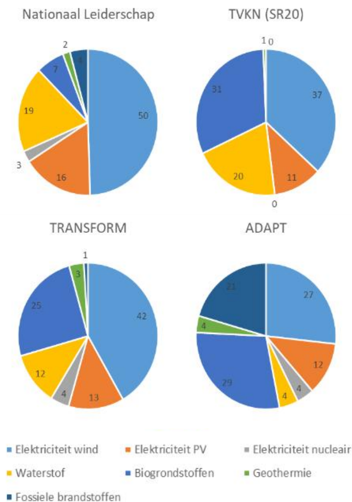
Figuur 3.1. Per scenario het percentage van de belangrijkste bronnen van energiebehoefte in 2050.
