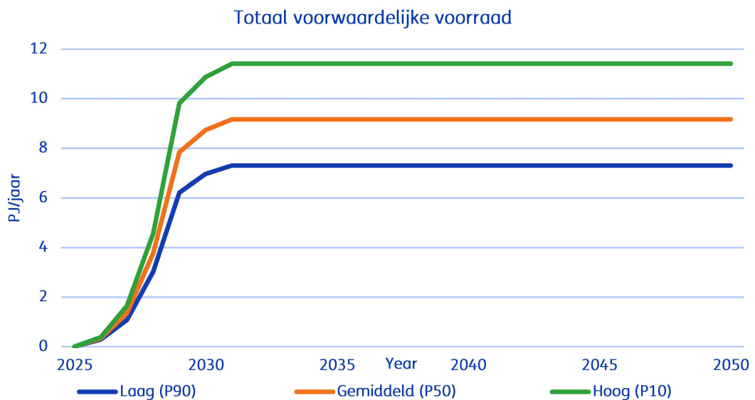
Figuur 6.7. Totaal voorwaardelijke aardwarmte aanbod tot 2050. Dit productieprofiel is opgebouwd uit alle aardwarmteprojecten die een SDE++ subsidie toegekend hebben. Deze projecten kunnen binnen een startvergunning of toewijzing zoekgebied liggen.
