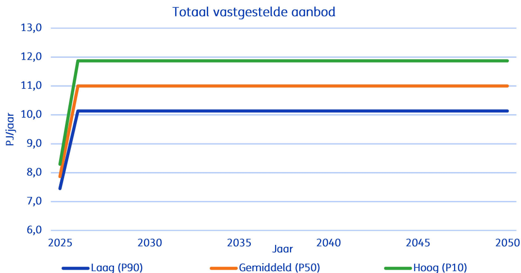
Figuur 6.6. Totaal vastgestelde aardwarmte aanbod. Dit productieprofiel is opgebouwd uit huidige en toekomstige productie van aardwarmteproductie-installaties in zowel start- als vervolgvvergunningen en installaties die nog in de opstartfase zitten.
