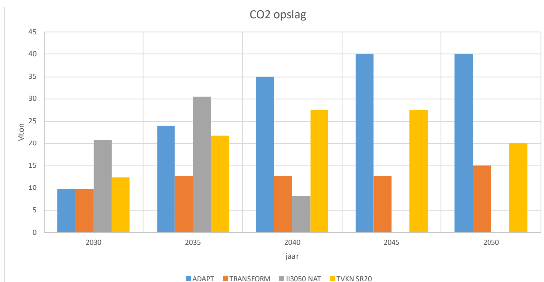
Figuur 3.2. Per scenario de behoefte aan CO 2 -opslag (Mton). Alleen in het scenario Nationaal Leiderschap (II3050 NAT) daalt de opslagbehoefte naar 0.
