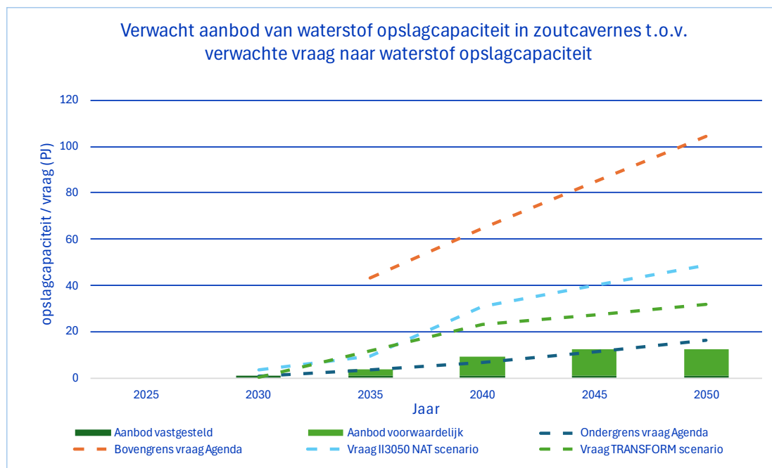
Figuur 8.1: Het verwachte aanbod van ondergrondse waterstof opslagcapaciteit in zoutcavernes tegen de verwachte vraag naar waterstofopslag in de periode 2030 – 2050. De boven- en ondergrens van de vraag zijn afgeleid uit de Nationale Agenda Ondergrondse Waterstofopslag.
