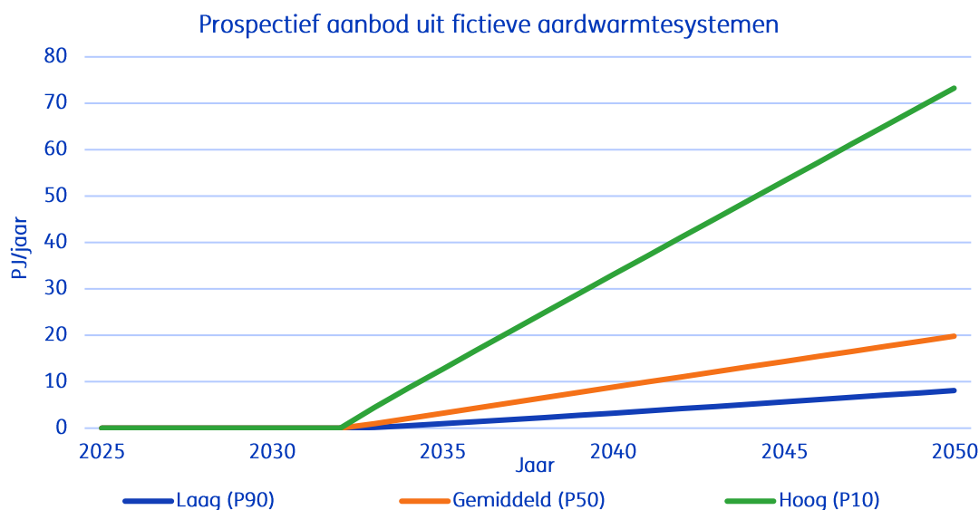
Figuur 6.9. Prospectief aardwarmte aanbod tot 2050. Dit productieprofiel is gemaakt op basis van fictieve aardwarmtesystemen. Dit zijn systemen die nog niet binnen een project of vergunning zijn gedefinieerd, en liggen daarom per definitie buiten een aardwarmtevergunning.
