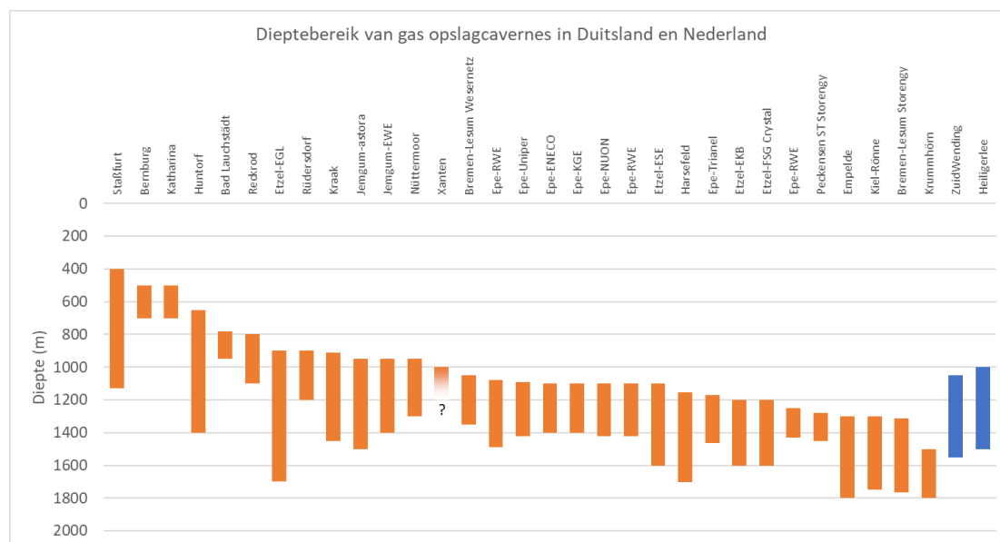
Figuur 8.5. Overzicht van het dieptebereik van opslagcavernes in Duitsland en Nederland. De twee blauwe staven representeren de bestaande Nederlandse gasopslag cavernes. De bron voor gegevens over Duitse cavernes is LBEG 2023, Untertage-Erdgasspeicherung in Deutschland (LBEG, 2024).
