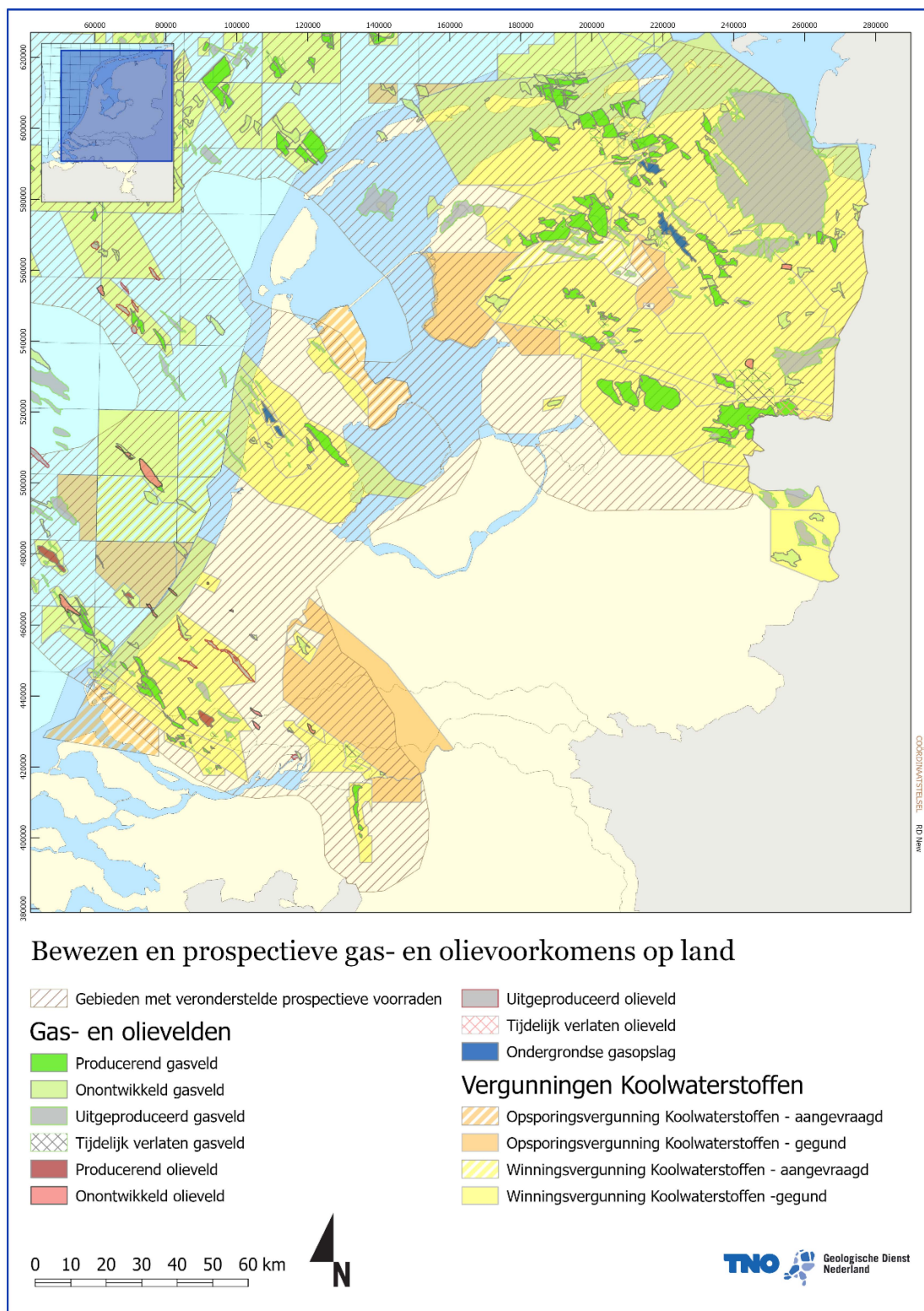
Figuur 4.3. Overzichtskartaal bewezen en prospectieve gas- en olievoorkomens op land (TNO DINO database).
