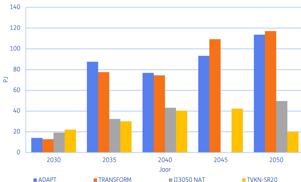
Figuur 6.4. Vraag naar aardwarmte tot 2050 volgens de vier onderzochte energiescenario's. In het II3050NAT scenario worden geen cijfers gegeven voor het jaar 2045.
