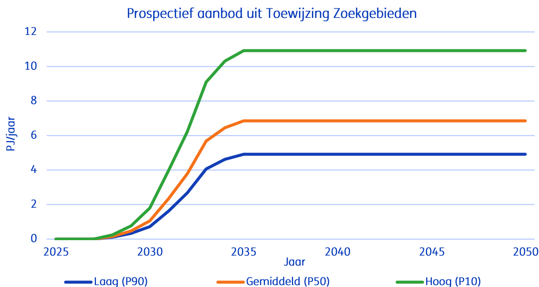
Figuur 6.8. Prospectief aardwarmte aanbod tot 2050. Dit productieprofiel is opgebouwd uit alle aardwarmte-projecten binnen een toewijzing zoekgebied die geen SDE++ toekenning hebben.
