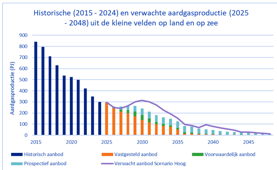
Figuur 4.5. Gerealiseerde (2015 - 2024) en verwachte (2025 - 2048) productie van aardgas uit de kleine velden op land volgens het Midden en Hoog scenario (Ministerie van Klimaat en Groene Groei, 2024). De gerealiseerde productie is exclusief productie uit het Groningen gasveld.
