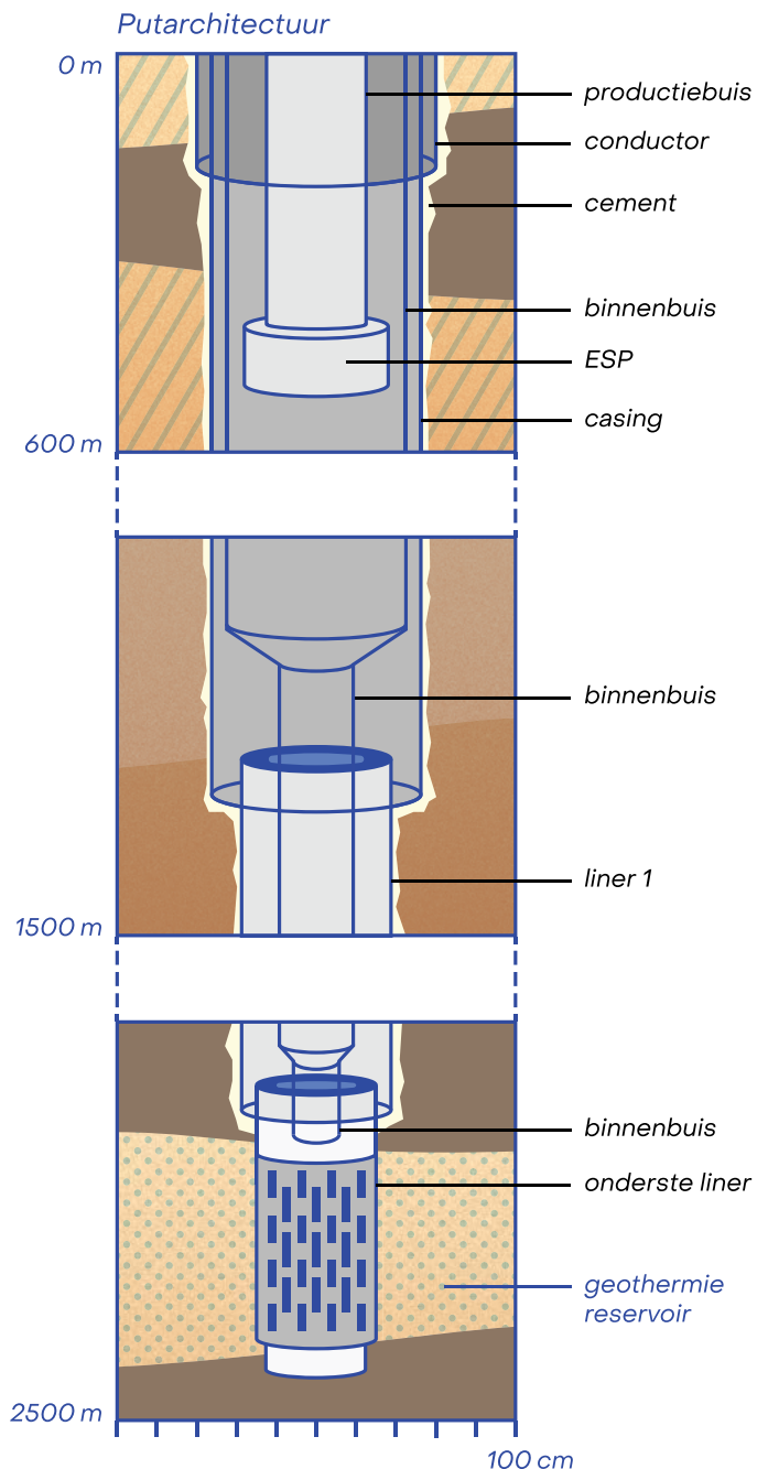
Figuur 2: Schematische weergave van de verbuizing van een geothermieput, volgens de Industriestandaard Duurzaam Putontwerp. De vermelde dieptes zijn voorbeelddieptes; dit is locatiespecifiek en verschilt per aardwarmtewinning.
