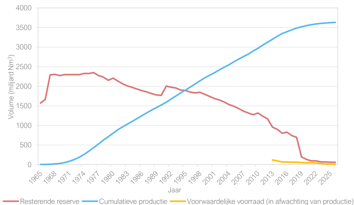
Figuur 1.2 Aardgasreserves en cumulatieve productie (1 januari 2026).
