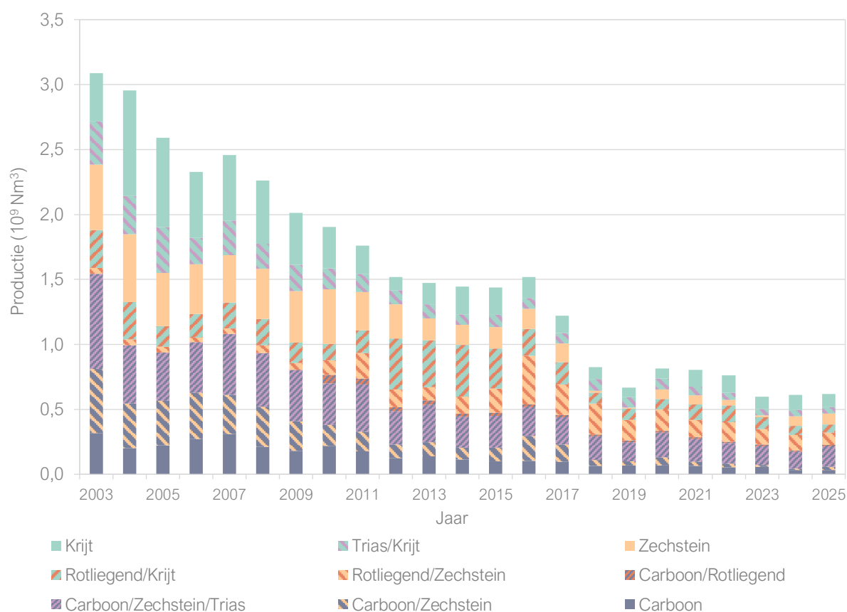
Figuur 3.2 Gasproductie op land, per reservoir (exclusief gasveld Groningen, Rotliegend en Trias reservoirs).
