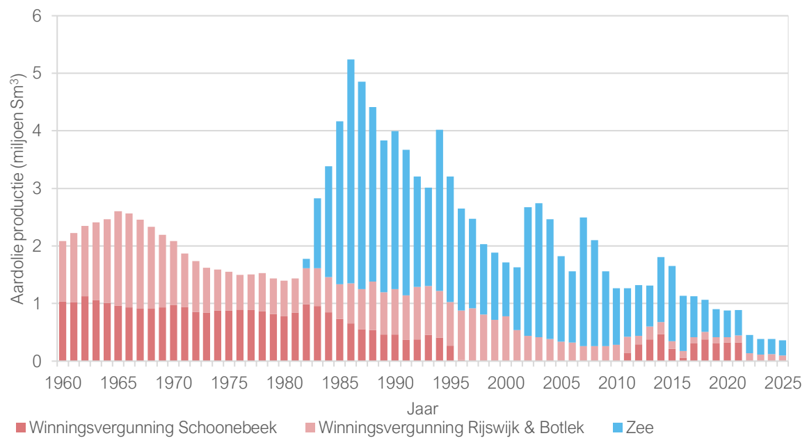
Figuur 3.6 Cumulatieve Aardolieproductie 1960 – 2025. Onderliggende gegevens zijn te vinden in Excel overzicht tabblad D. N.B. De aardolieproductie wordt in dit figuur weergegeven voor gasvelden op land en op zee. Deze waarden kunnen licht afwijken van die in Hoofdstuk 3.3 en 3.4, waar de productie per vergunning wordt gepresenteerd.
