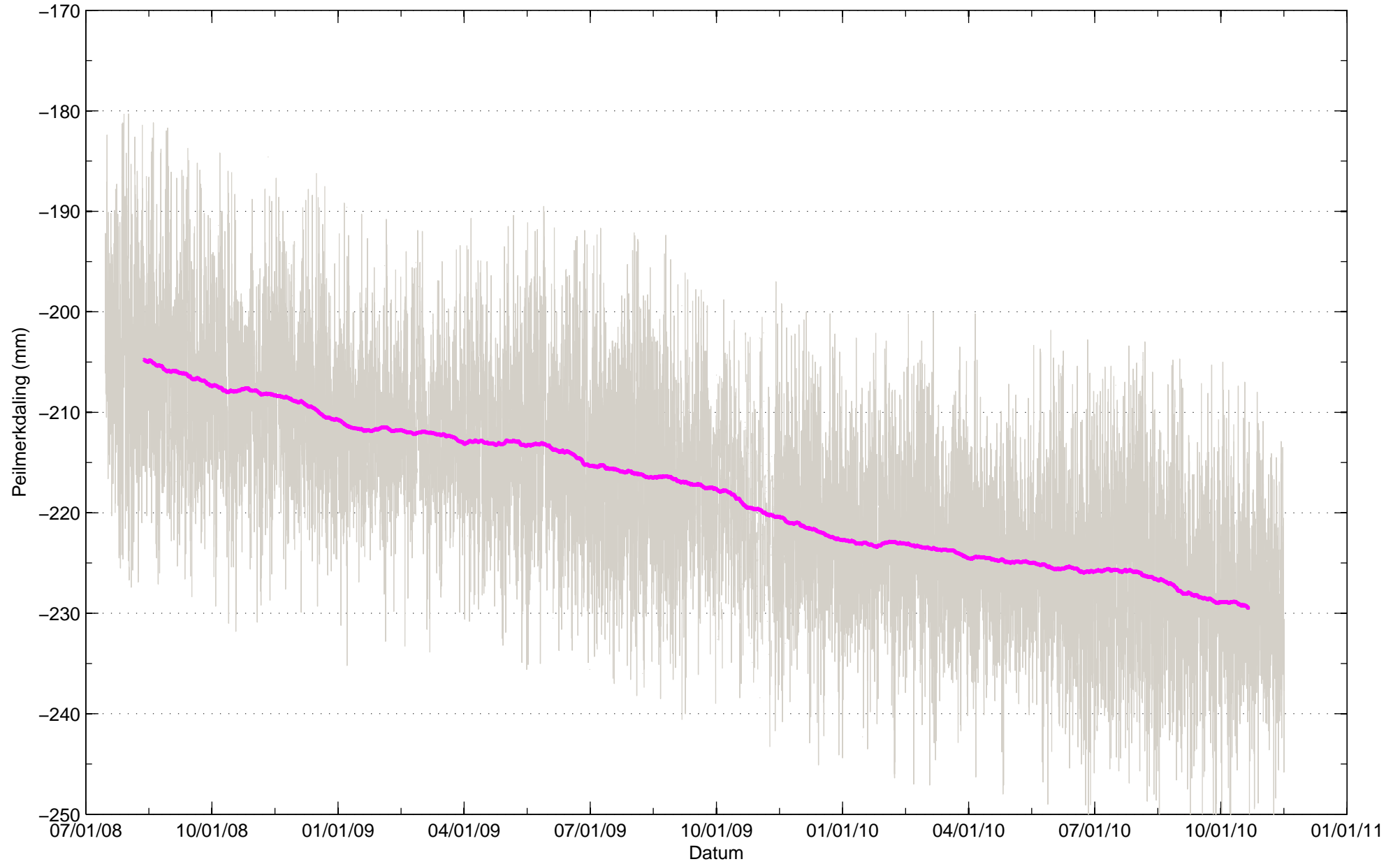
Bodemdaling Leeuwarden West GPS station HRL7 Resultaten uit permanente GPS meting
